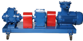
减速机结构 Coupling Drive
